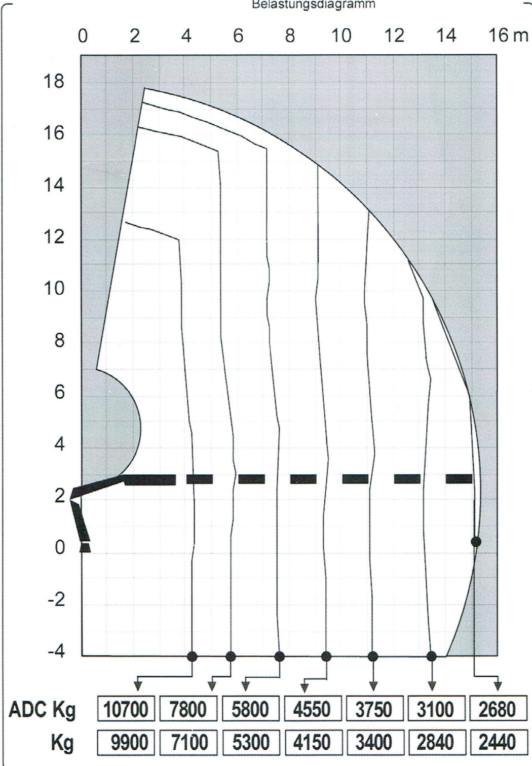
Belastungsdiagramm
